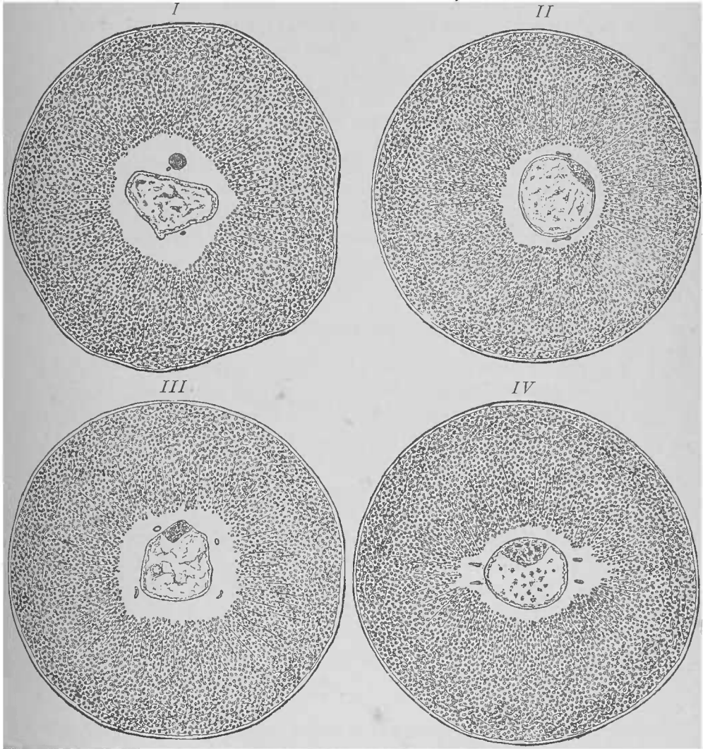
FIG. 144. — Le quadrille des centres , d'après Fol (VII, 14).
