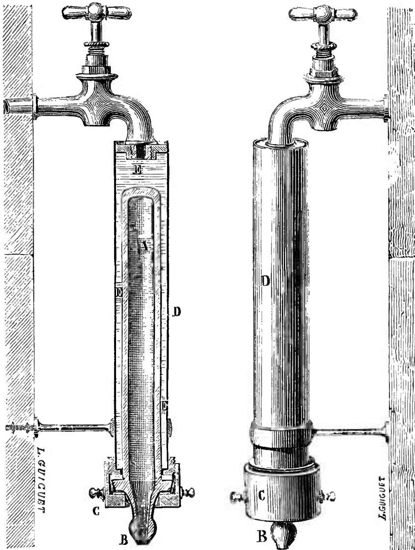
Fig. 101. — Profil et coupe d'un filtre Chamberland pour la purification des eaux potables.
