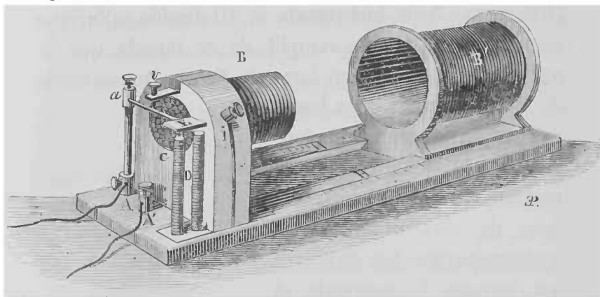
FIG. 71. — Appareil volta-faradique de Du Bois-Reymond.
