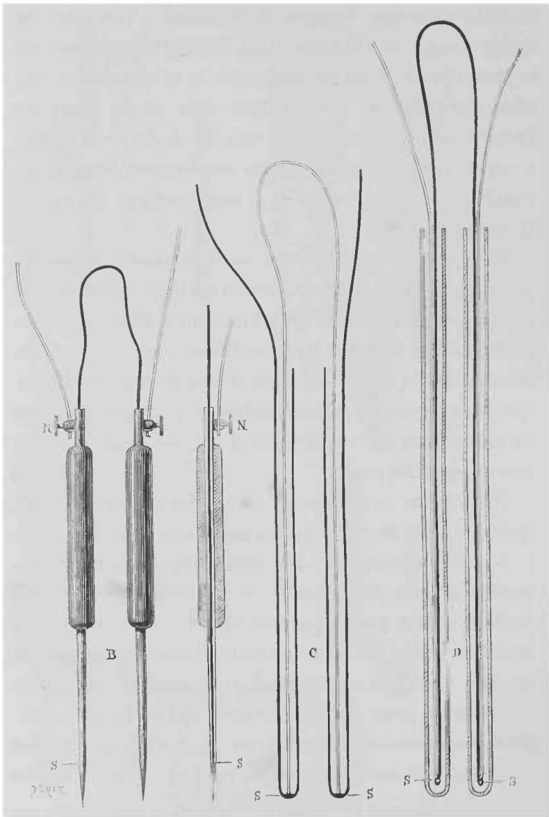
FIG. 101. — Sondes thermo-électriques de d'Arsonval.
