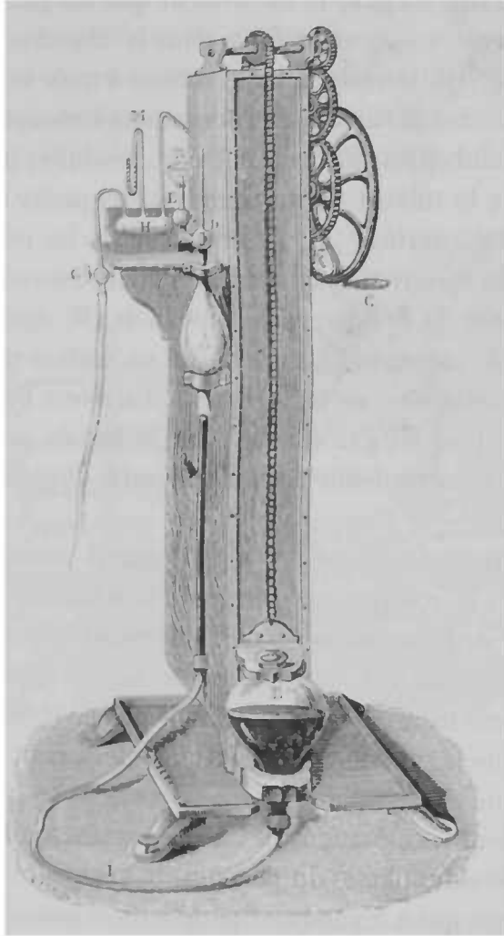
FIG. 66. — Pompe à mercure.
