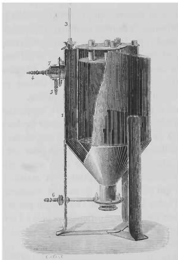
FIG. 106. — Appareil de d'Arsonval pour obtenir une température constante.
