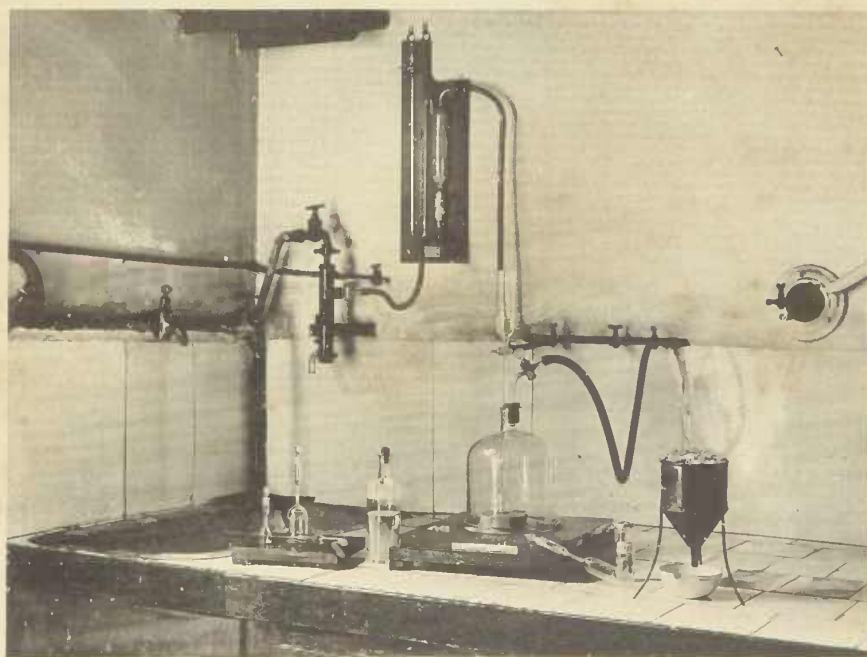
Fig. 1. Boîte à échantillons d'eaux marines. — Fig. 2. Bouteille Richard en descente. Fig. 3. Bouteille Richard en montée. — Fig. 4. Mesure de la densité des échantillons d'eaux et de fonds marins.
