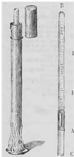
Fig. 46. — Lacto-butyromètre de E. Marchand.
