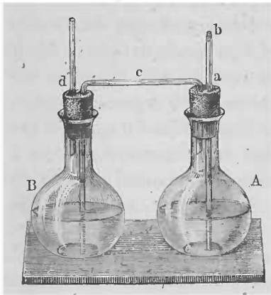
Fig. 35. — Dosage du sucre de l'urine par fermentation.
