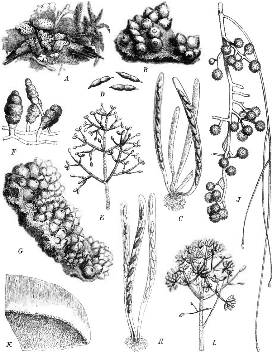
Fig. 236. A–F Hypomyces ochraceus (Pers.) Tul. A Stromata, nat. Gr.; B reife Fruchtkörper (20/1); C Schläuche (380/1); D Sporen (350/1); E Conidienträger (ca. 130/1); F Chlamydosporen (ca. 200/1). — G–J H. chrysospermus (Bull.) Tul. G Fruchtkörper, vergr.; H Schläuche (380/1); J Chlamydosporen und Conidien (380/1). — K H. viridis (Alb. et Schw.) Berk. et Br., Habitus des Pilzes auf Lactaria (3/1). — L H. rosellus (Alb. et Schw.) Tul., Conidienträger (ca. 130/1). (K Original; das übrige nach Tulasne.)
