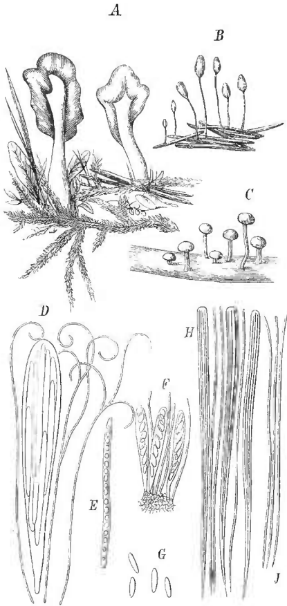
Fig. 138. A, D, E Spathularia clavata (Schaeffer) Saccardo. A Habitusbild; D Schläuche und Paraphysen; E Spore. — B, F, G Mitrula cucullata (Batsch) Fries. B Habitusbild; F Schläuche und Paraphysen; G Sporen. — C, H, J Vibrissa truncorum (Albertini et Schwein.) Fries. C Habitusbild; H Schläuche und Paraphysen; J Sporen. (A—C nat. Gr., D, E 500/1, F 400/1, H, J 350/1.) (Sämtlich n. d. Natur.)
