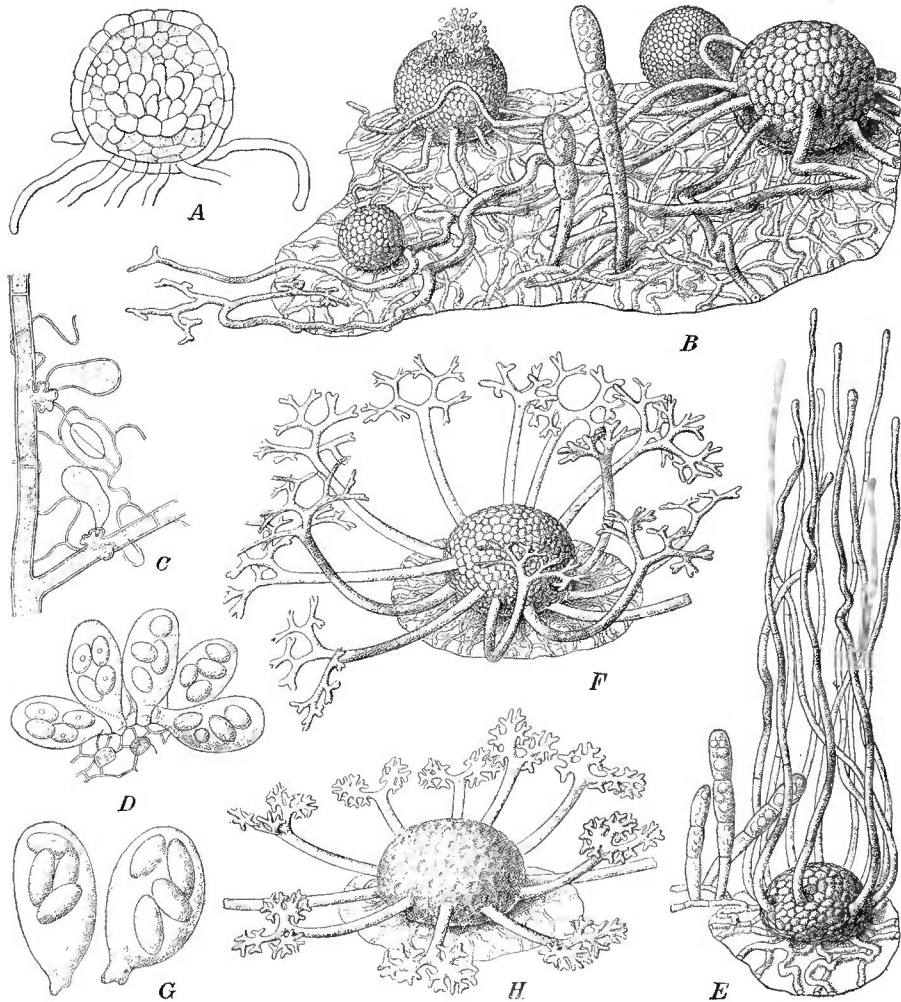
Fig. 229. A, B Erysiphe communis (Wallr.) Link. A junger Fruchtkörper mit Ascogonium, im Querschnitt (400/1); B Fruchtkörper und Conidien (ca. 175/1). — C, D E. Heraclei DC. C Haustorien (400/1); D Schläuche (200/1). — E E. Aspyrali DC., Fruchtkörper mit Conidienträger (ca. 175/1). — F, G Microsphaera Berberidis (DC.) Lévl. F Fruchtkörper (ca. 175/1); G Schläuche (350/1). — H M. Alni (DC.) Wint., Fruchtkörper (200/1). (A, C, D nach De Bary; das übrige nach Tulasne.)
