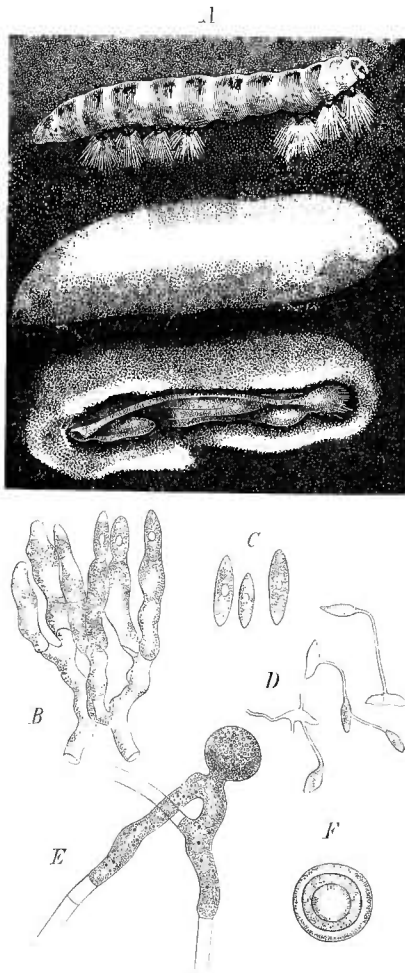
Fig. 124. Entomophthora sphaerosperma Fresen. A durch den Pilz getötete Raupen in verschiedenen Stadien der Entwicklung des Pilzes; B verzweigte Basidienträger; C Conidien; D secundäre und tertiäre Conidien; E Dauersporenbildung; F reife Dauerspore. (A nat. Gr., B, D 300/1, C 650/1, E, F 350/1.) (A—D nach Brefeld; E, F nach Nowakowski.)
