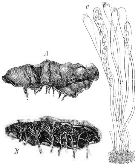
Fig. 143. Rhizina inflata (Schäffer) Saccardo. A Fruchtkörper von vorn; B derselbe von unten; C Schläuche und Paraphysen. (A, B nat. Gr., C etwa 400/l.) (A, B nach der Natur; C nach Tulasne.)
