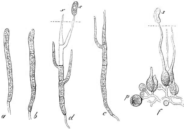
Fig. 40. a-d quergeteilte Basidien von Auricularia auricula Judae . — f geteilte Basidien von Exidia spiculosa (390/4). (Nach De Bary.)
