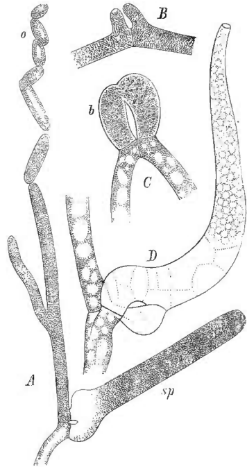
Fig. 129. Dipodascus albidus Lagerheim. A Mycelast mit Conidien (a) und einem jungen Sporangium (sp); B erste Anlage der Gameten; C Copulation; D reifer Sporenschlauch. (A etwa 200/1, B–D 500/1.) (Nach Lagerheim.)
